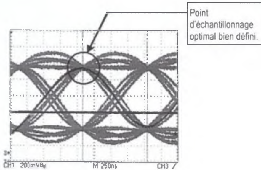
Figure 12-3. Diagramme en œil idéal
