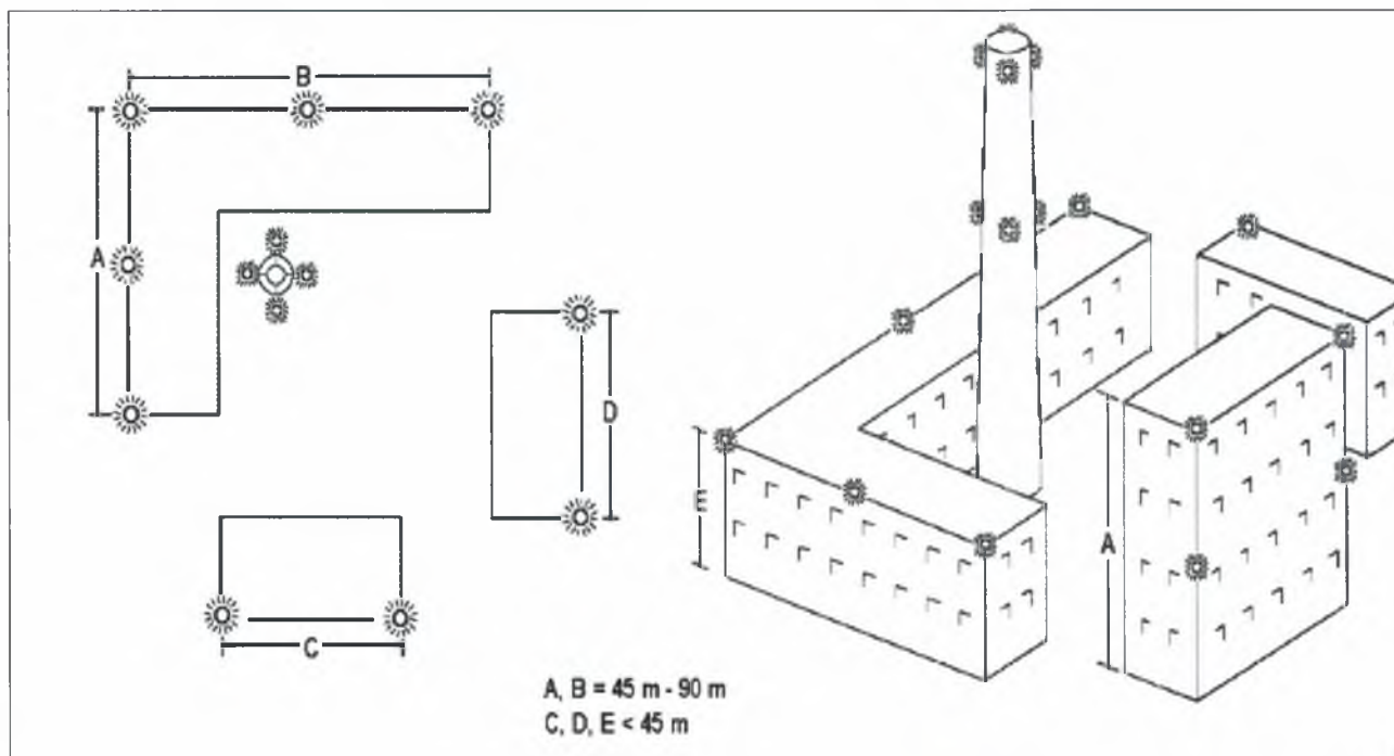
Figure 3. Balisage lumineux des constructions
