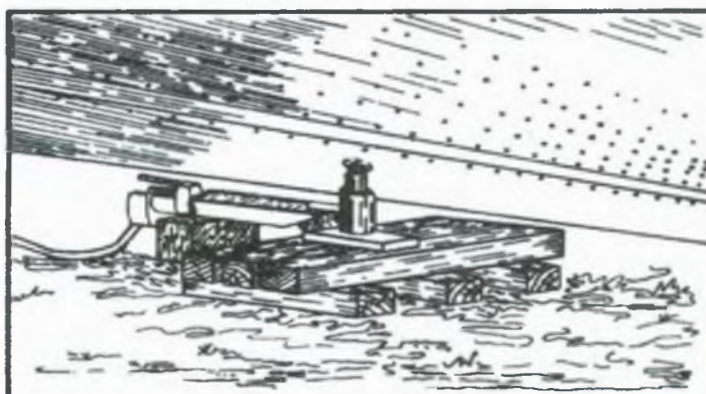
Figure 3 Bases pour vérins et sacs pneumatiques de levage en terrain mou
