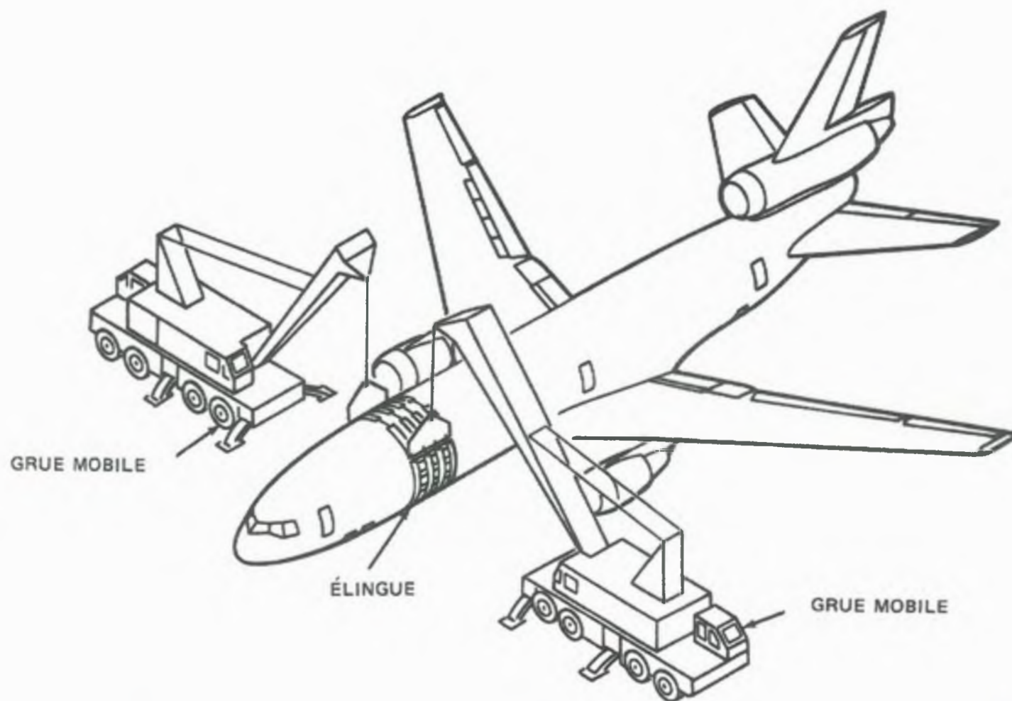
Figure 6 Illustration de la méthode de levage de la pointe avant à l'aide de grues mobiles
