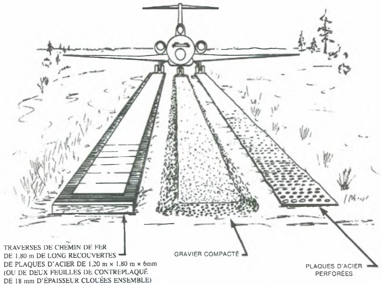
Figure 2 Différents types de surfaces préparées
