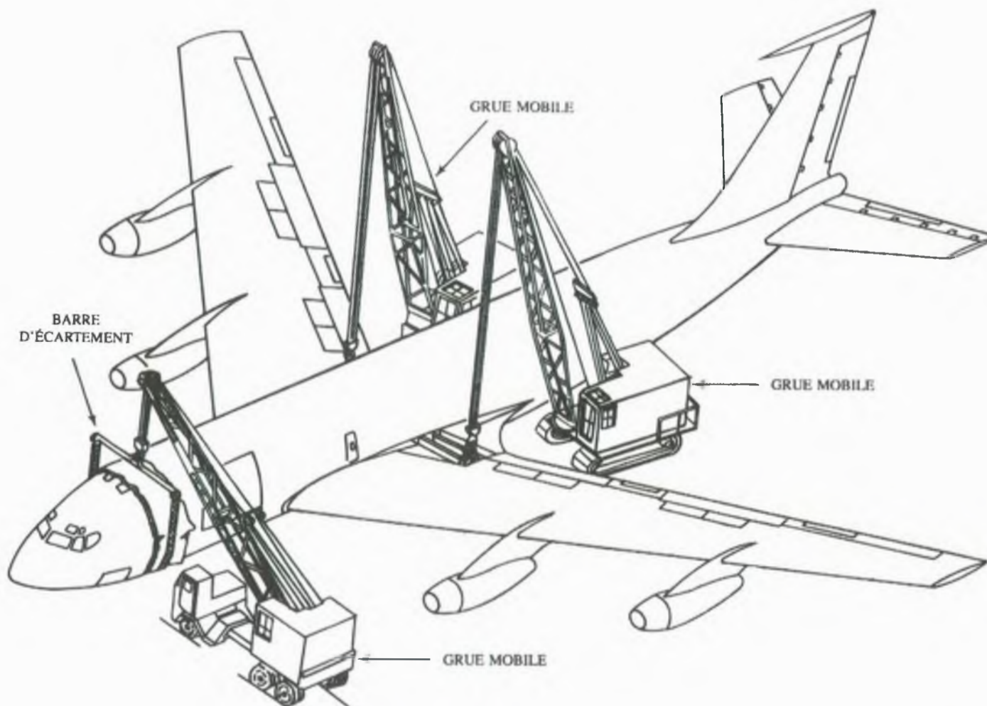
Figure 7 Illustration de la méthode de levage d'un avion au moyen de grues mobiles
