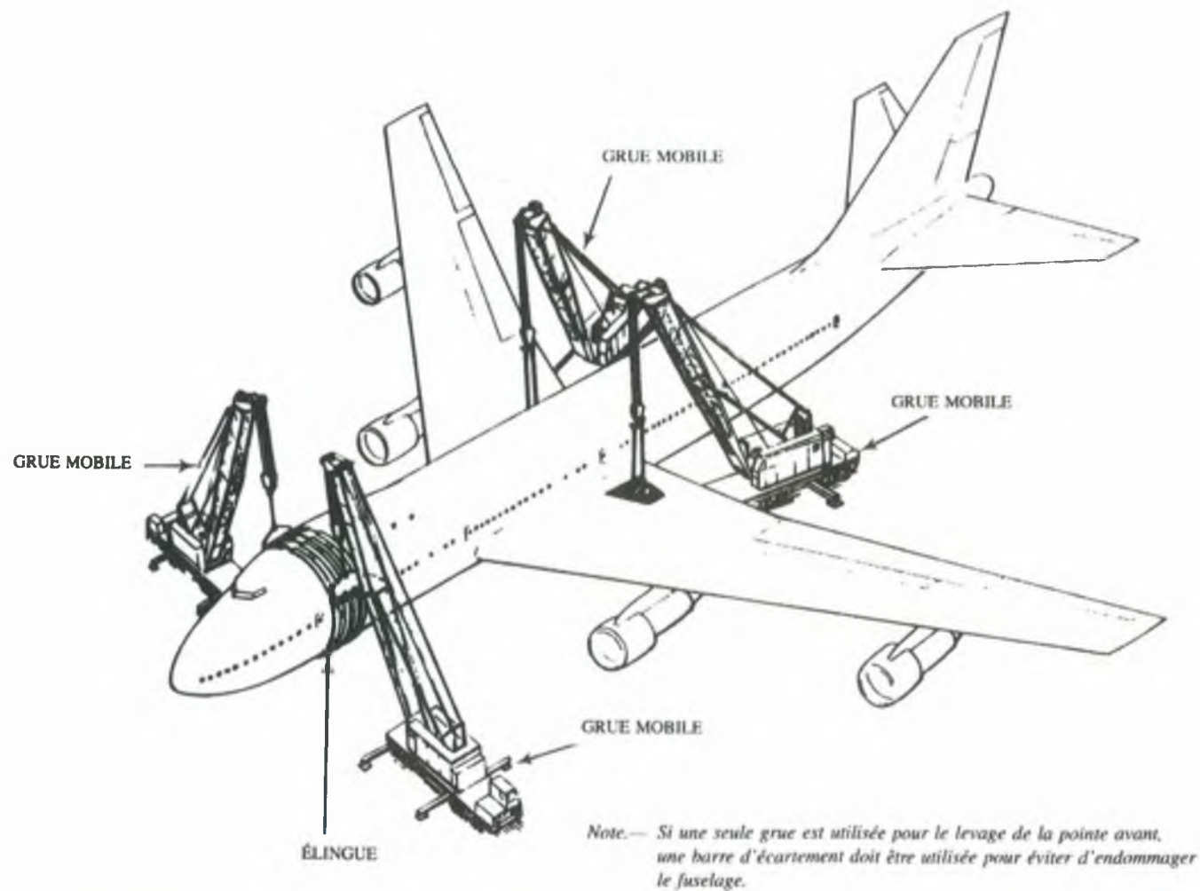
Figure 8 Illustration de la méthode de levage d'un gros-porteur au moyen de grues mobiles
