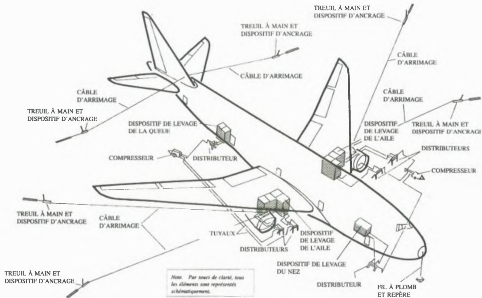
Figure 9 Disposition typique du matériel
