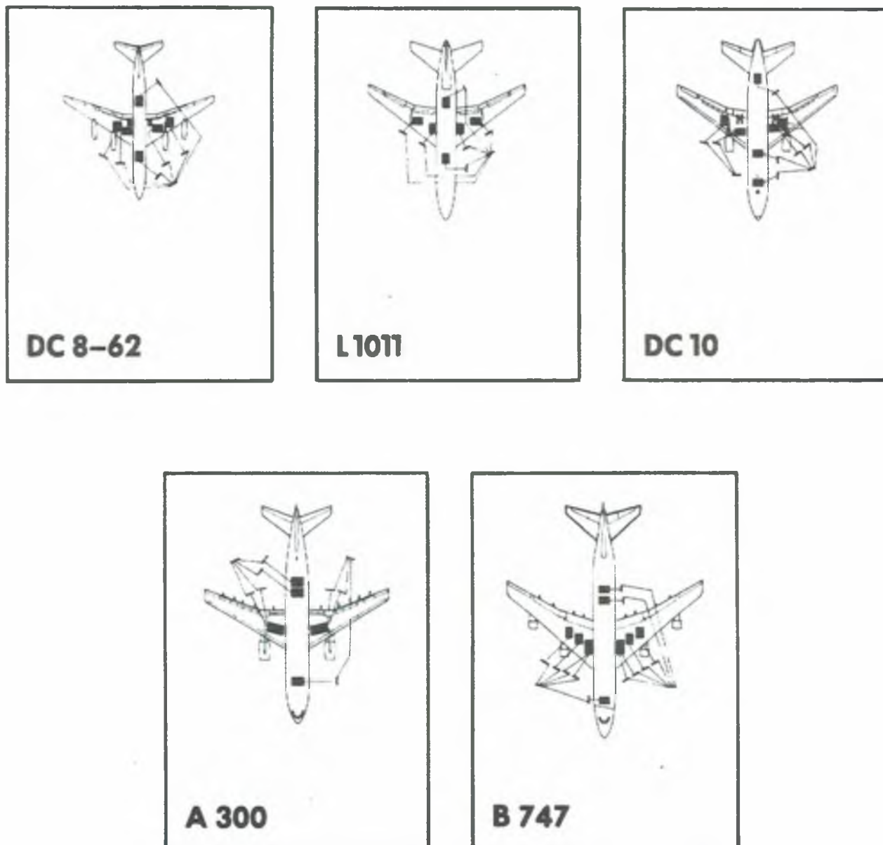
Figure 10 Disposition typique des sacs pneumatiques de levage
