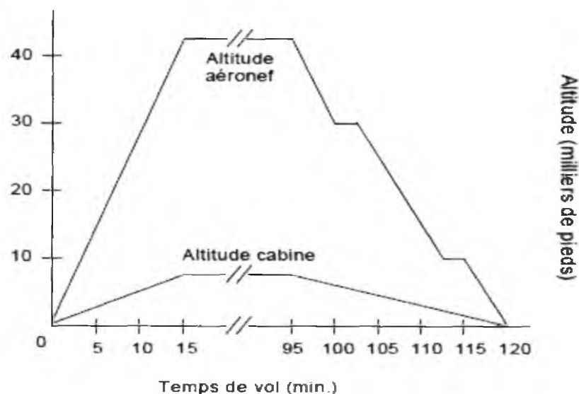
Figure II-1-4. Altitude de l'aéronef et altitude cabine pour un aéronef commercial pendant un vol type 1
