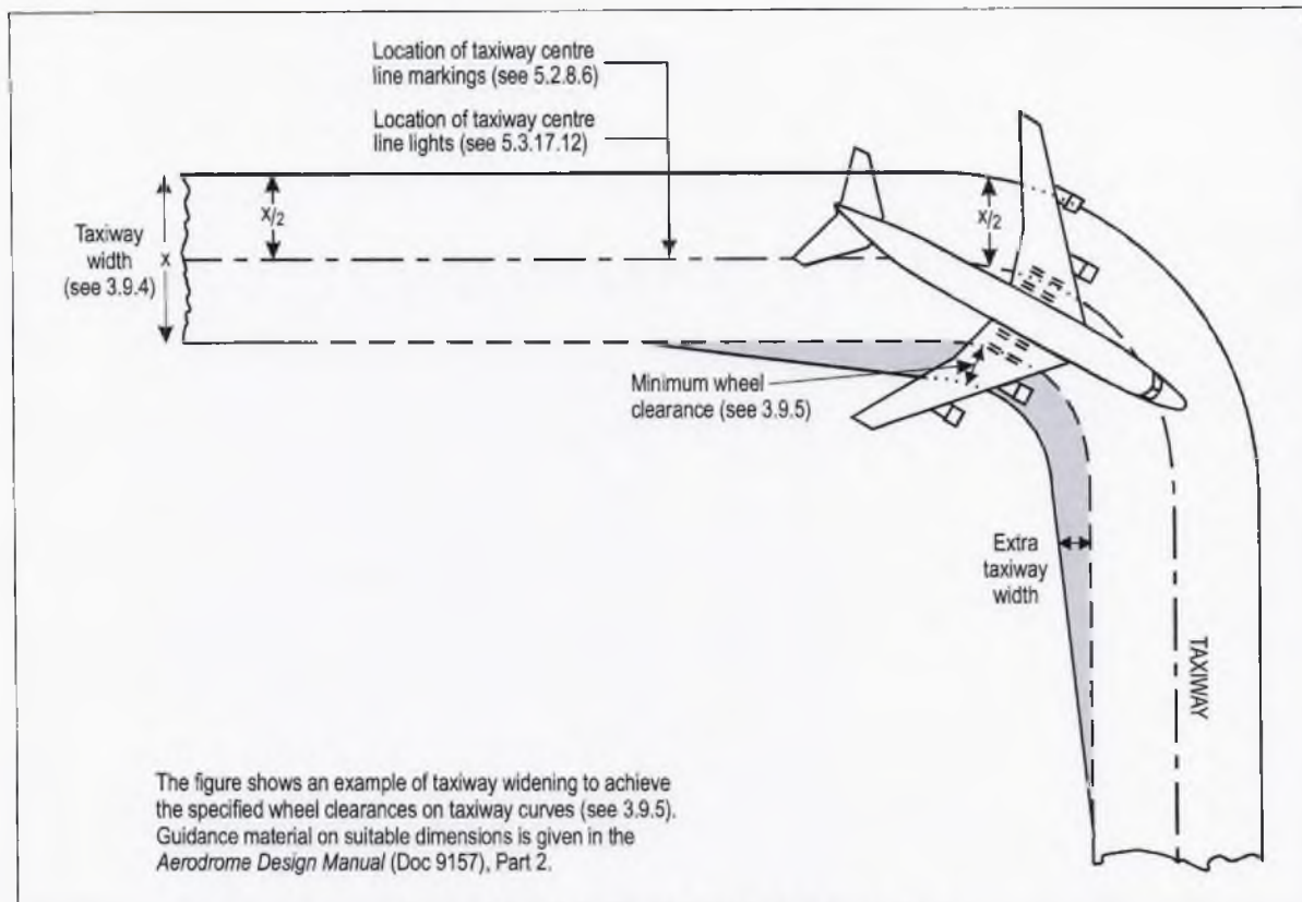
Figure 3-2. Virage de voie de circulation
