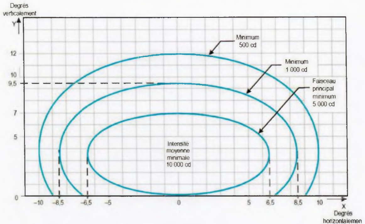
Figure A2-9. Diagramme isocandela des feux de bord de piste avec 45 m de largeur de piste (lumière blanche)
