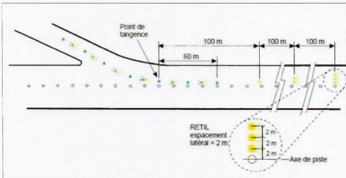
Figure 5-25. Feux indicateurs de voie de sortie rapide (RETIL)
