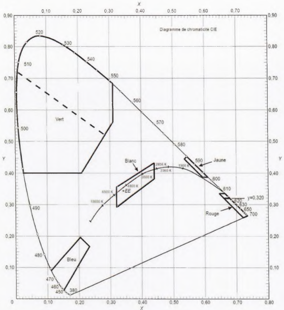
Figure A1-1b. Couleurs des feux aéronautiques à la surface (feux semi-conducteurs)
