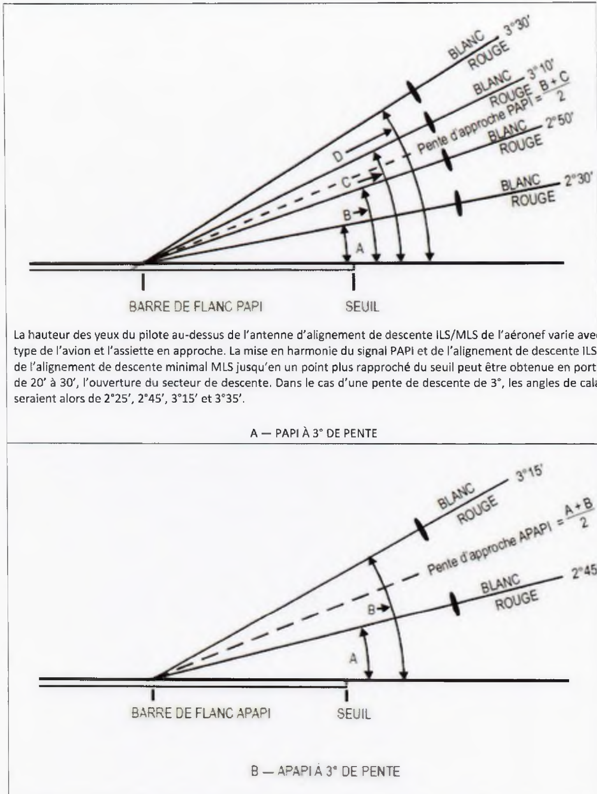
Figure 5-20. Faisceaux lumineux et calage en site d'un PAPI et d'un APAPI
