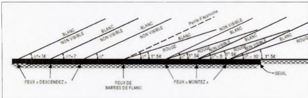
Figure 5-18. T-VASIS et AT-VASIS — Faisceaux lumineux et calage angulaire en site
