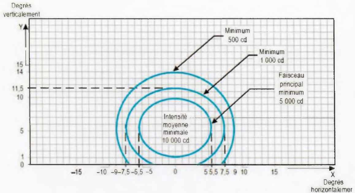
Figure A2-2. Diagramme isocandela des feux de barrette latérale d'approche (lumière rouge)
