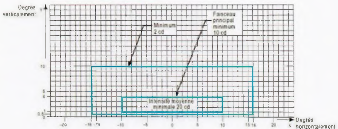
Figure A2-14. Diagramme isocandela des feux d'axe de voie de circulation (espacement de 7,5 m), REL, feux de barre d'entrée interdite et de barre d'arrêt dans les sections courbes, valant pour des conditions donnant lieu à une portée visuelle de piste inférieure à 350 m
