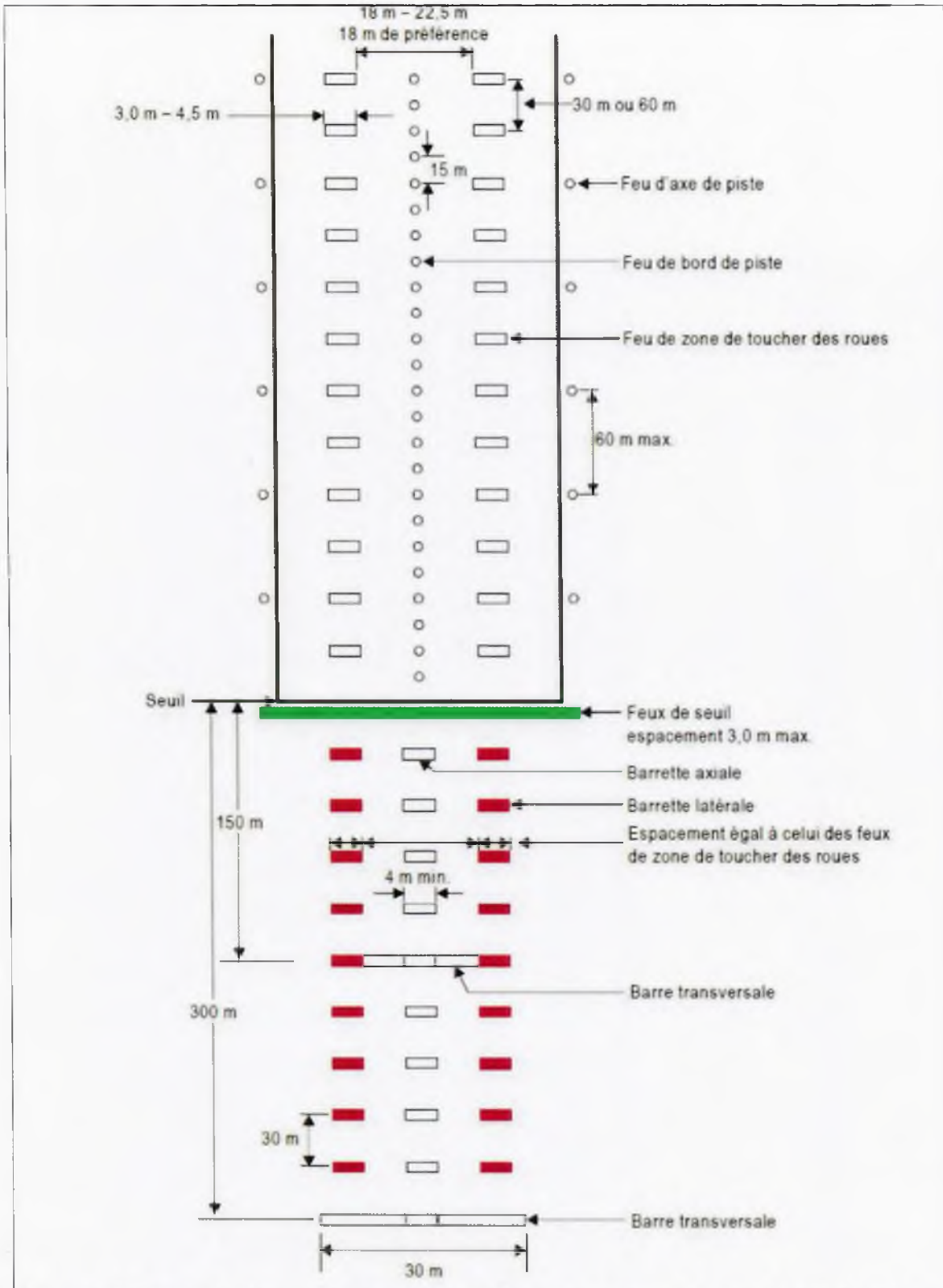
Figure 5-14. Balisage lumineux de la piste et des 300 derniers mètres de l'approche pour les pistes avec approche de précision des catégories II et III
