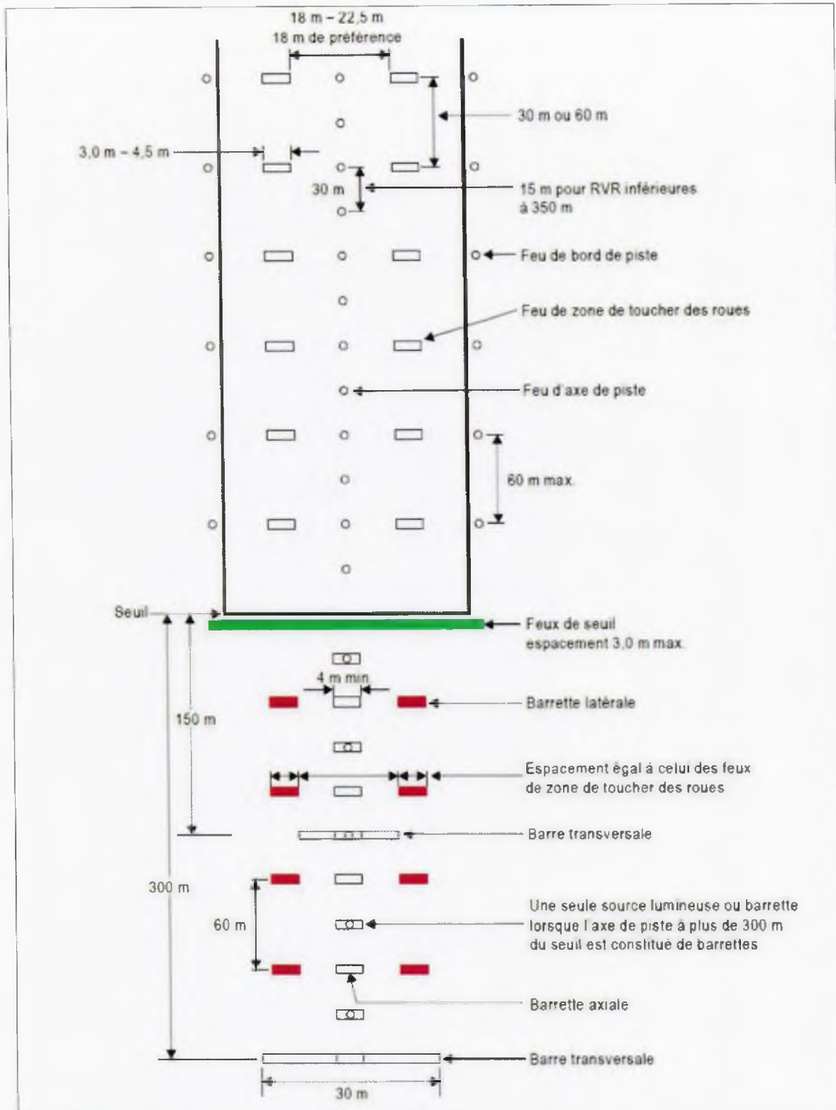
Figure 5-15. Balisage lumineux de la piste et des 300 derniers mètres de l'approche pour les pistes avec approche de précision des catégories II et III quand le niveau de fonctionnement spécifié comme objectif d'entretien au Chapitre 10 peut être démontré
