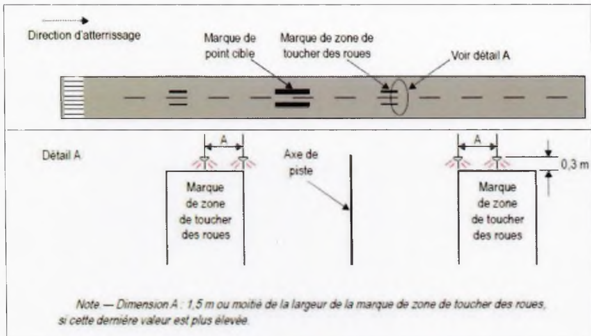
Figure 5-24. Feux simples de zone de toucher des roues
