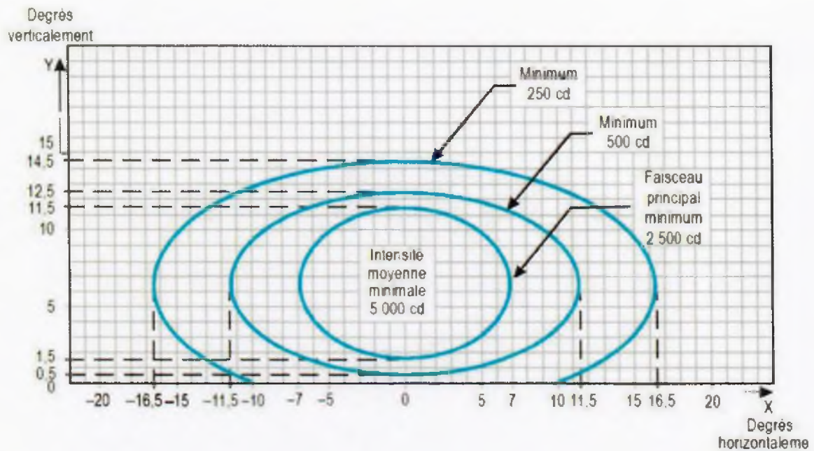
Figure A2-1. Diagramme isocandela des feux de ligne axiale et des barres transversales d'approche (lumière blanche)
