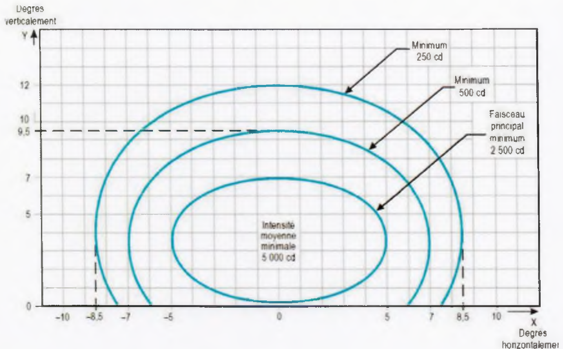
Figure A2-5. Diagramme isocandela des feux de zone de toucher des roues (lumière blanche)
