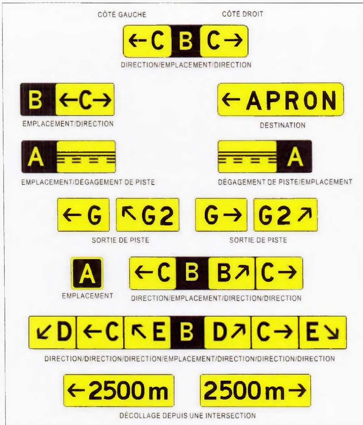
Figure 5-31. Panneaux d'indication
