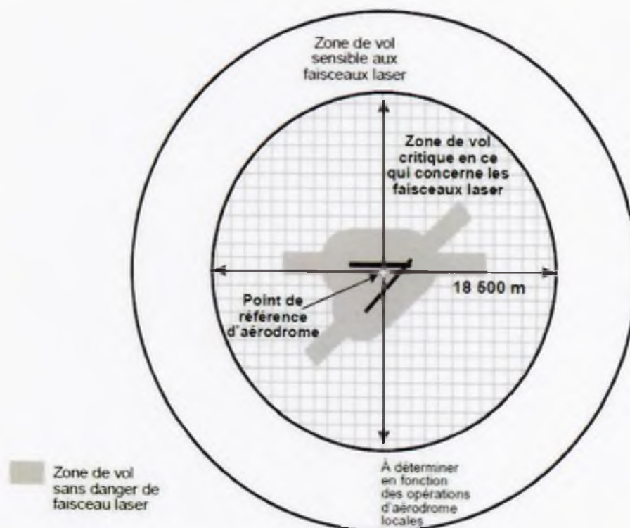
Figure 5-11. Zones de vol protégées
