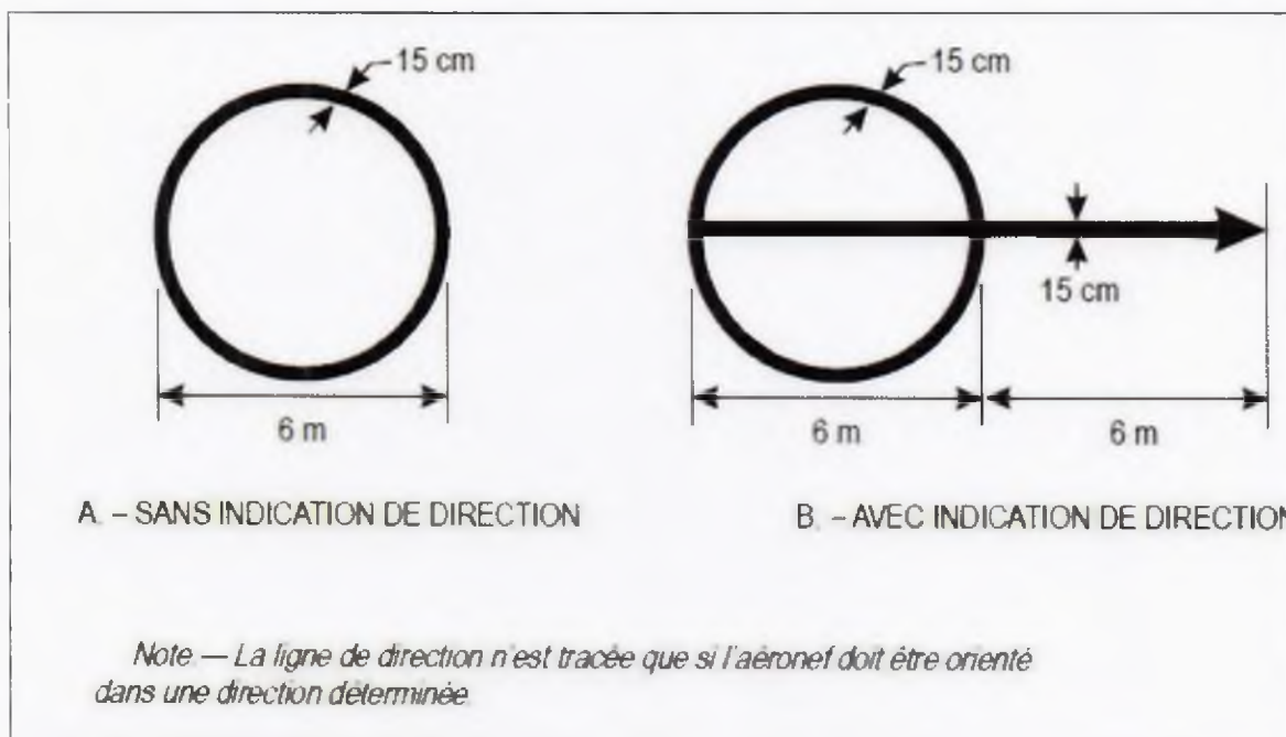
Figure 5-9. Marques de point de vérification VOR d'aérodrome
