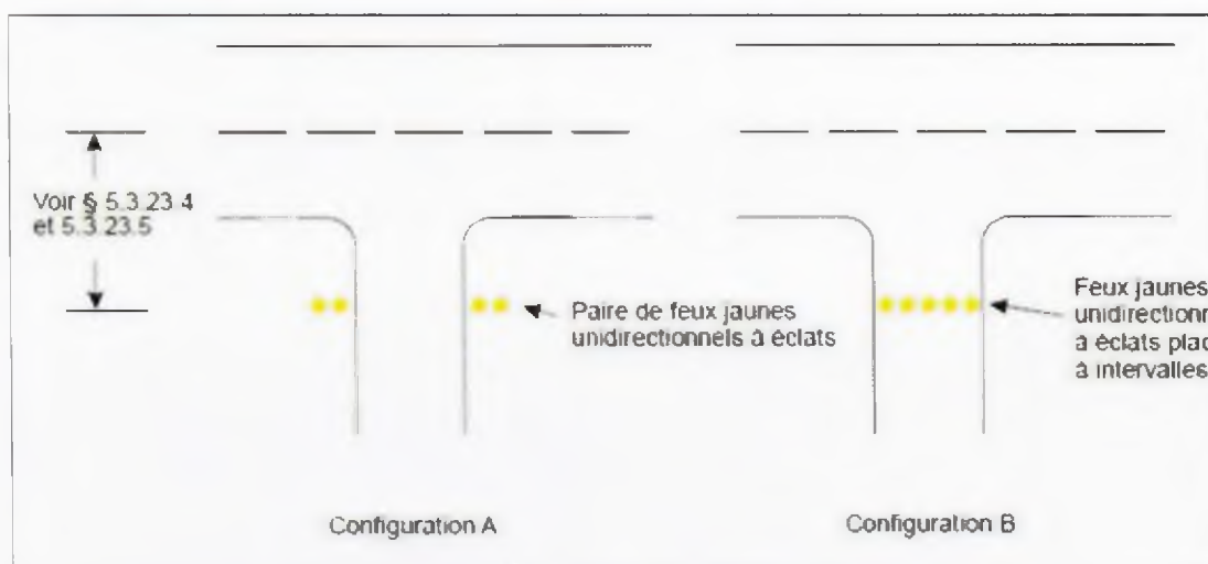
Figure 5-29. Feux de protection de piste
