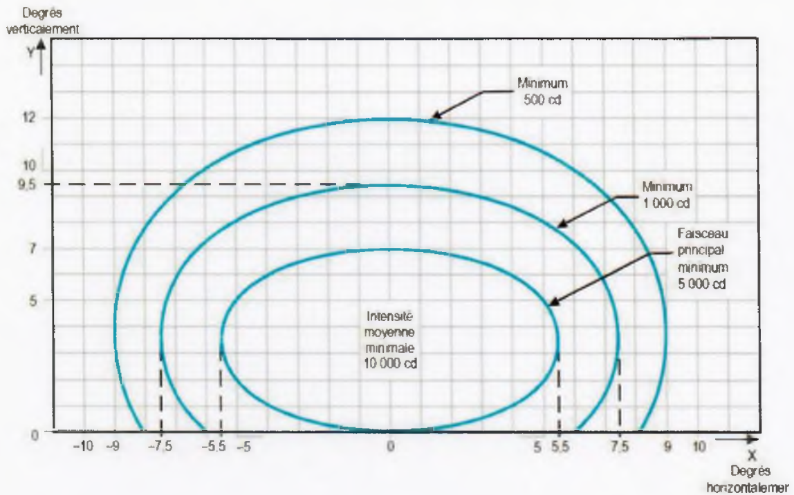
Figure A2-8. Diagramme isocandela des feux d'extrémité de piste (lumière rouge)
