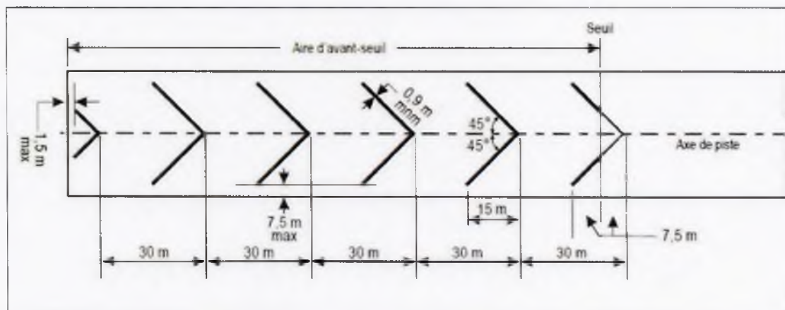
Figure 7-2. Marques d'avant-seuil
