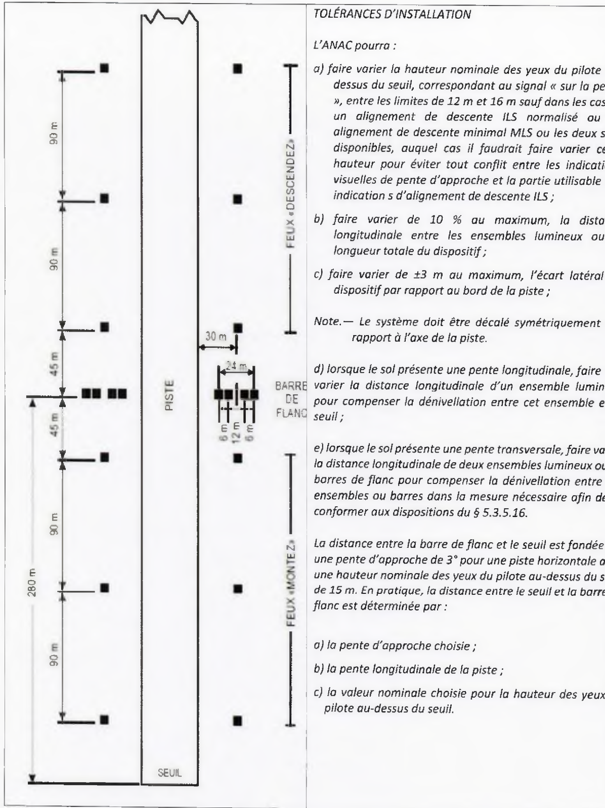
Figure 5-17. Emplacement des ensembles lumineux du T-VASIS
