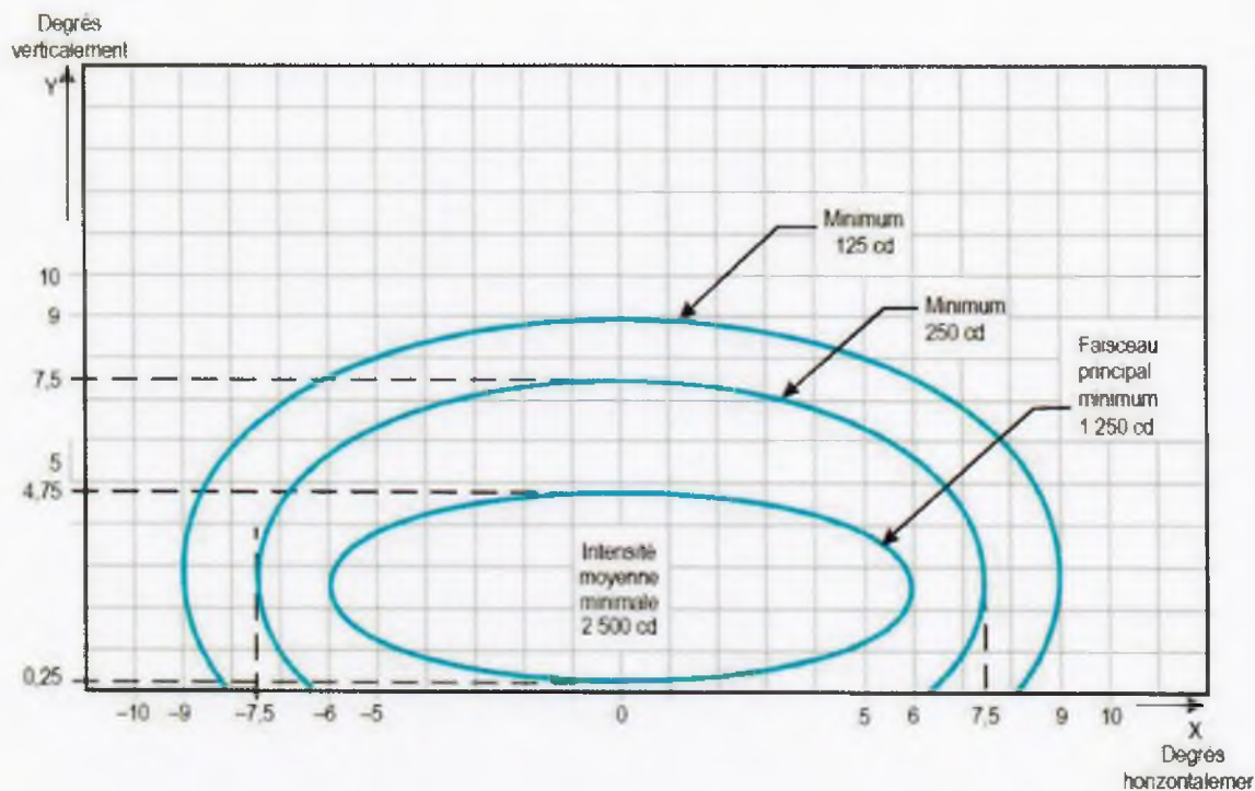
Figure A2-7. Diagramme isocandela des feux d'axe de piste avec intervalle longitudinal de 15 m (lumière blanche) et des feux indicateurs de voie de sortie rapide (lumière jaune)
