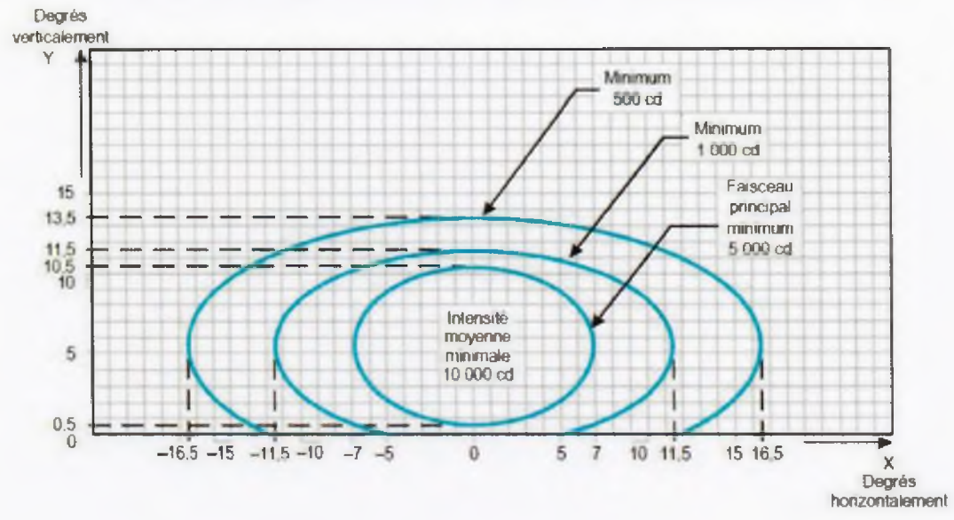
Figure A2-3. Diagramme isocandela des feux de seuil (lumière verte)
