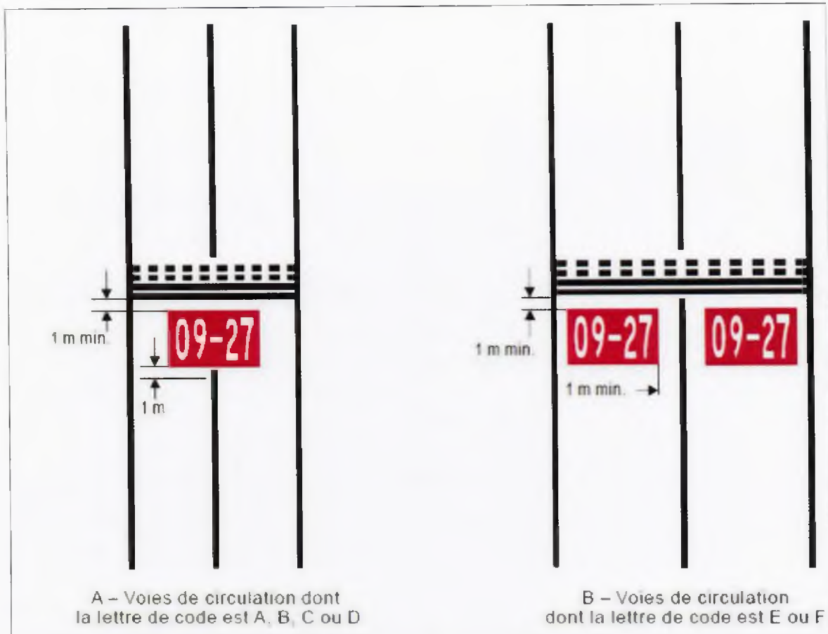
Figure 5-10. Marque d'obligation
