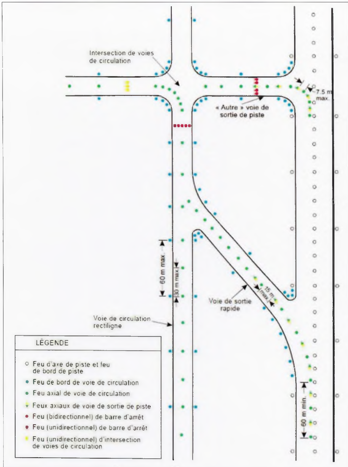
Figure 5-26. Balisage lumineux de voie de circulation
