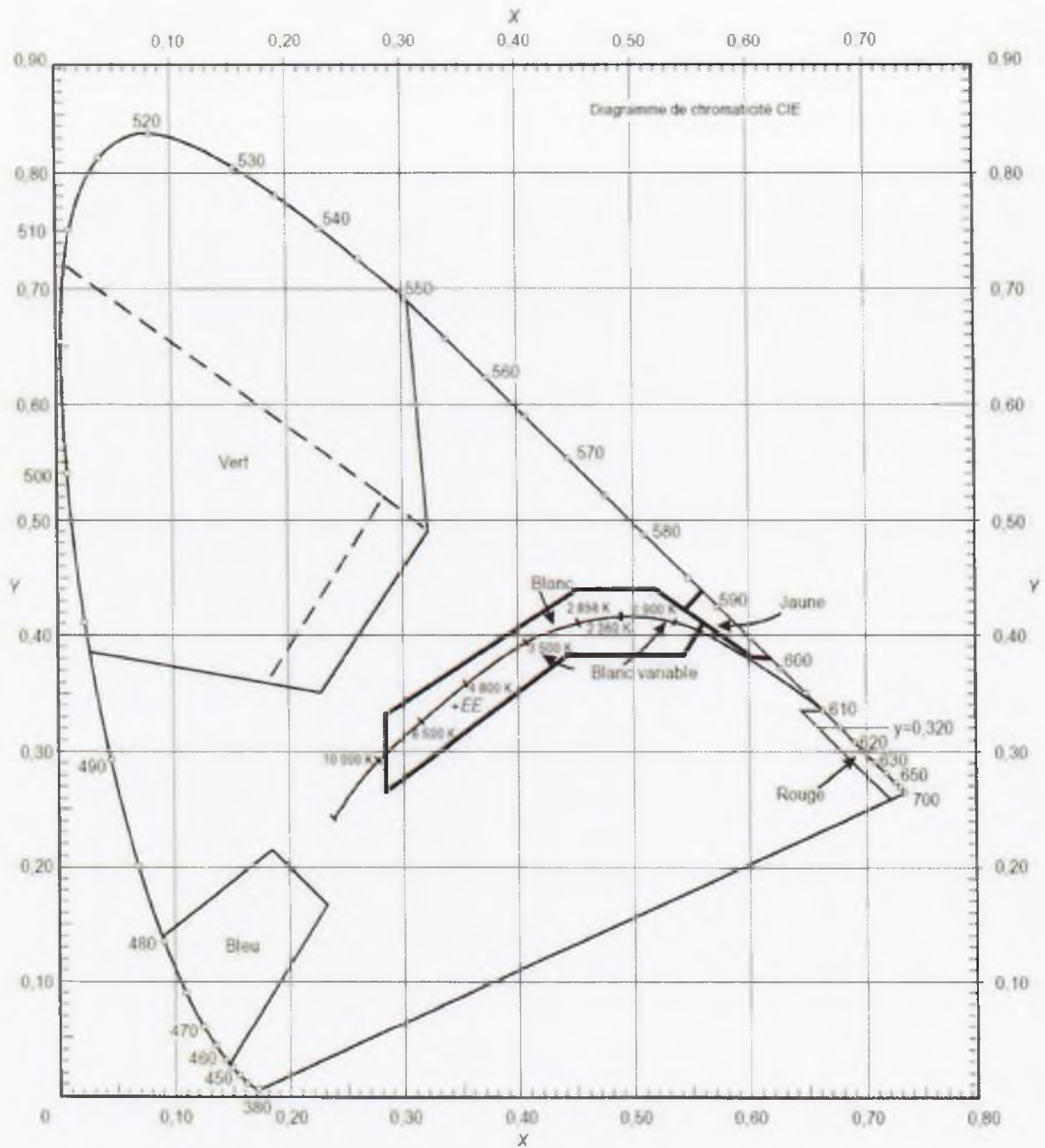
Figure A1-1a. Couleurs des feux aéronautiques à la surface (lampe à incandescence)
