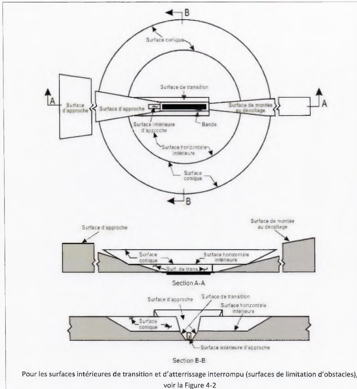
Figure 4-1. Surfaces de limitation d'obstacles
