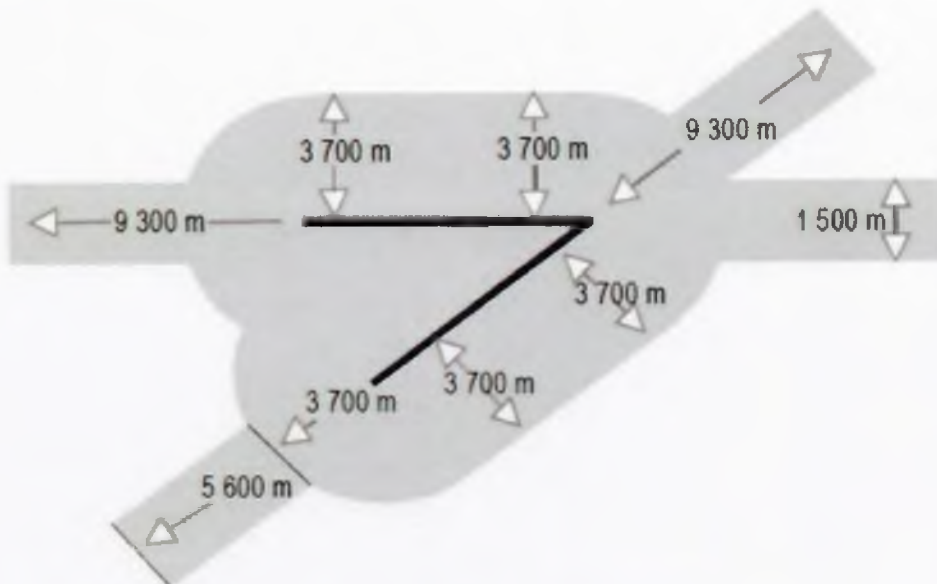
Figure 5-12. Zone de vol sans danger de faisceau laser pour pistes multiples
